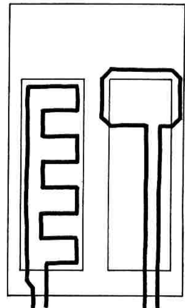
Falsch: a) Kabelkamm strahlt kein Magnetfeld ab b) Schleife ist zu klein
