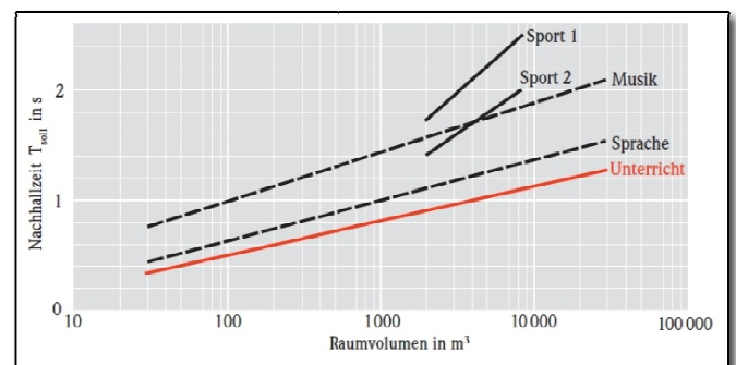
Abb. 2 – Sollnachhallzeit in Abhängigkeit von Raumgröße (nach DIN 18041)
