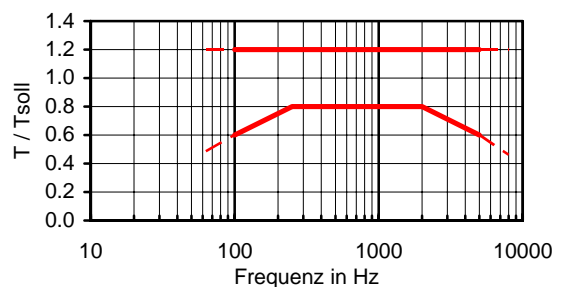
Abbildung 2 Toleranzbereich der empfohlenen Nachhallzeit in Abhängigkeit von der Frequenz für Sprache gemäss DIN 18041, Bild 2
