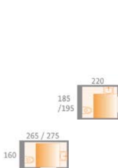
Flächenbedarf einer einseitig anfahrbaren Toilette mit Waschtisch oder Handwaschbecken
